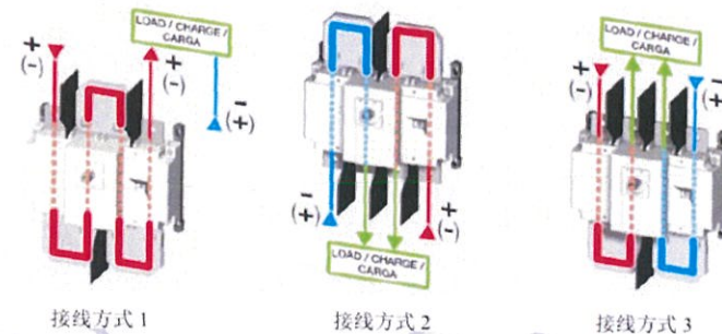
1000VDC 4P 外形接线图
