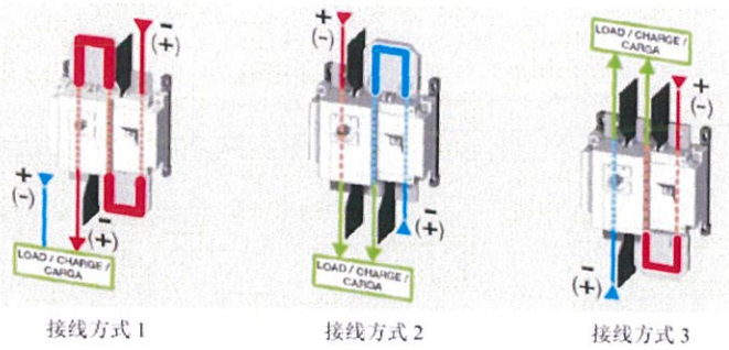
1000VDC 4P 外形接线图
