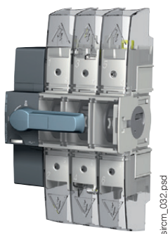
Accionamiento frontal directo
