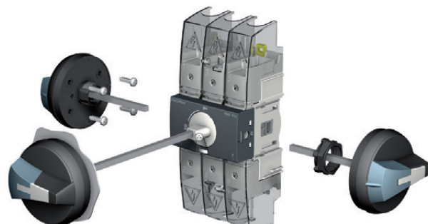
Accionamiento exterior parte frontal, lateral izquierdo o derecho
