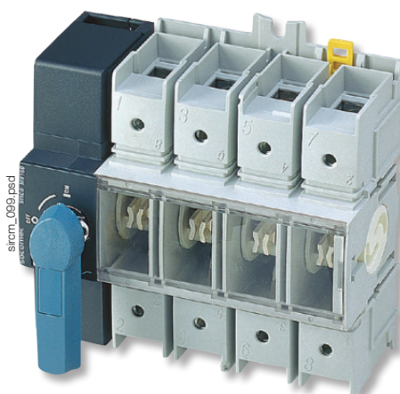
SIRCO MV de 4 polos mando directo
