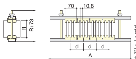
Inserto de 10 mm / 3 barras
