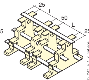
Tipo 2: Embarrados incluyendo 3 (o más) soportes SB E 44 con soportes intermedios duplicados.
