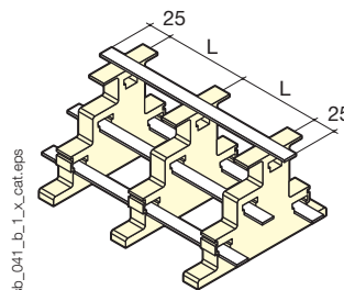
Tipo 1: Embarrados que incluyen 3 (o más) soportes SB E 44 a la misma distancia.
