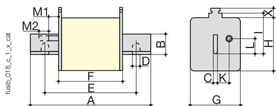
Dimensiones estándar (mm) según IEC 60269-2-1
