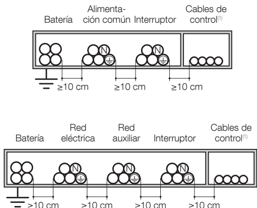
Instalación aceptable
