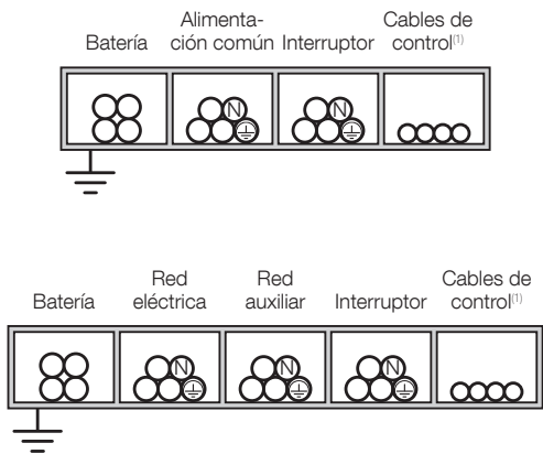
Instalación correcta
