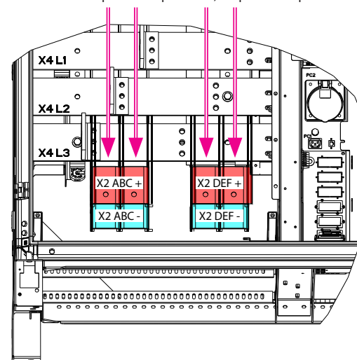
Batería compartida de forma flexible para 3 cajas de RANURAS de potencia
