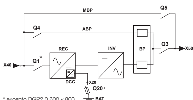
ENTRADA COMÚN DE RECTIFICADOR Y BYPASS
